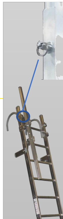
Echelle avec crochets Ø300 mm et crosse télescopique à gauche. Pour déployer la crosse tirer sur l'anneau.
